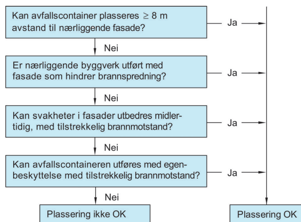
Fig. 63 b Flytskjema for å verifisere om plasseringen av oppsamlingsenhetene representerer fare for brannspredning
